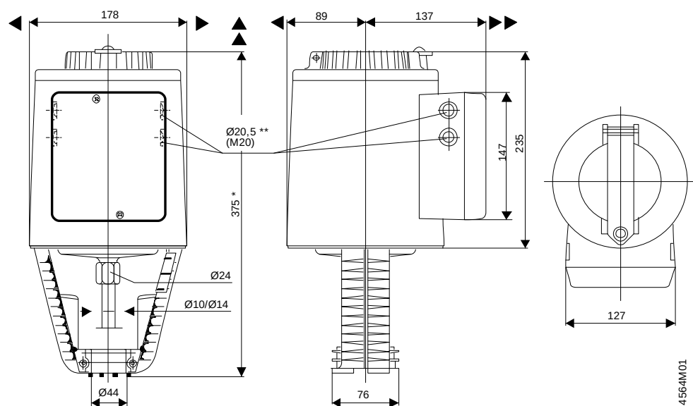
尺寸 (mm)
